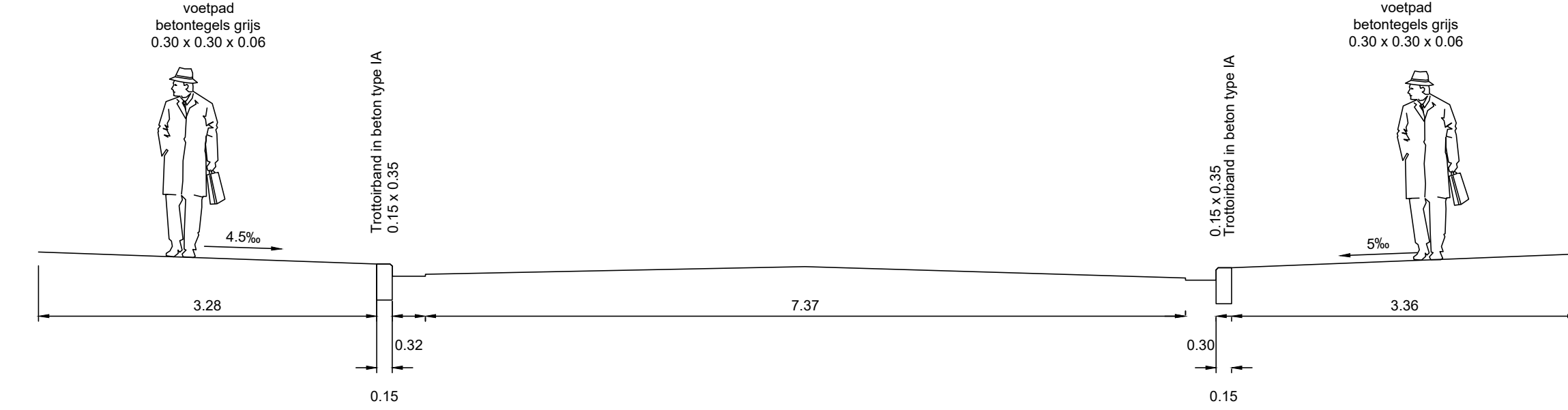
TYPE DWARSPROFIEL: A-A ontwerpen toestand schaal 1:100
